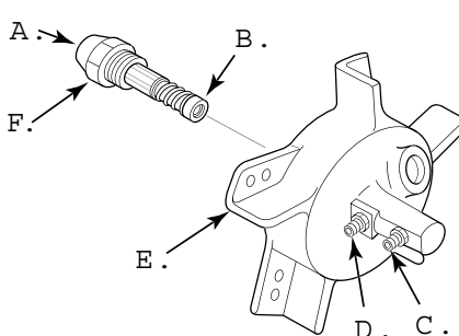
24. ábra - A fűvóka kiszerelése, 20/29/44 kW modellek
