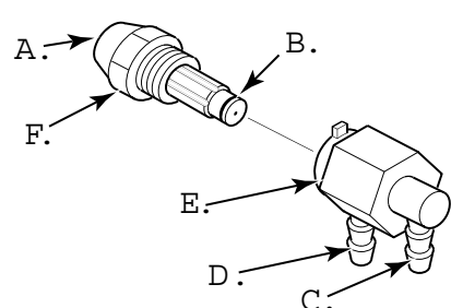
Figur 22 – Dyse og dysebøsning.
