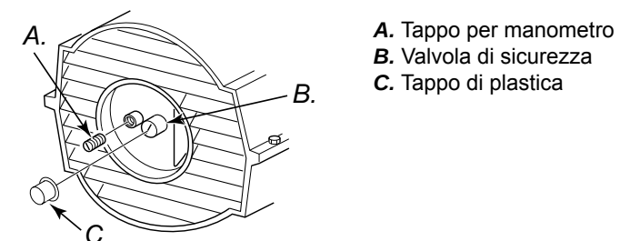
Figura 18 – Rimozione del tappo per manometro.
