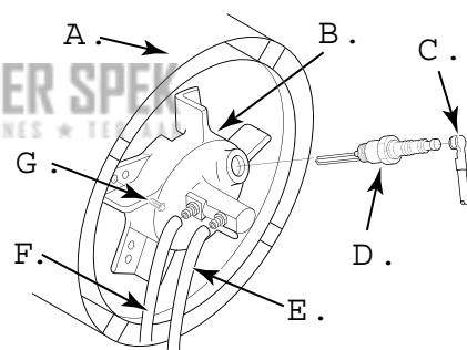
Figur 23 Fjernelse af Brndkammerhovedet, 20/29/44 kW.
