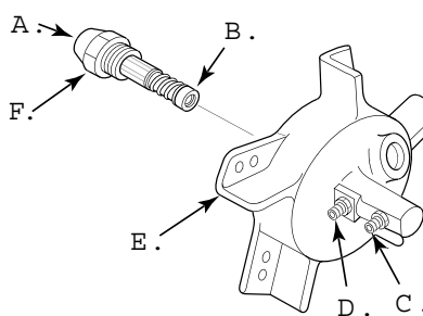
Kuva 24 – Suuttimen irrotus, mallit (vain mallit 20/29 ja 44 kW).
