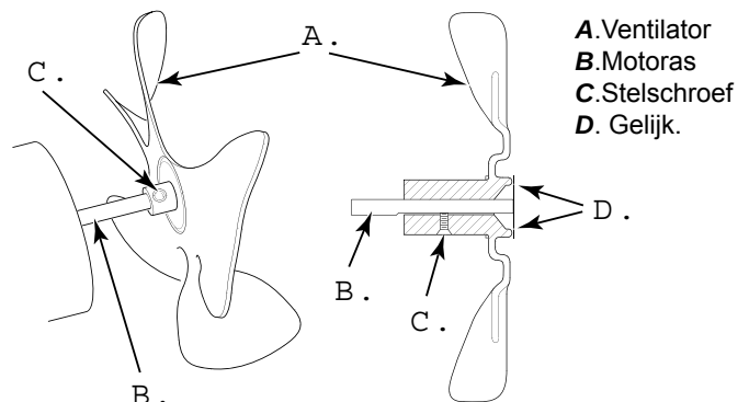
Figuur 29 – Plaats van ventilator, motoras en stelschroef.
