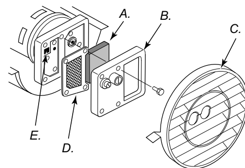
Rysunek 17 - Filtr wylotu powietrza, filtr wlotu powietrza i filtr włókninowy, modele 29 kW i 44 kW
