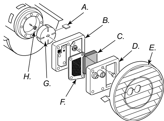
Figura 25 – Ubicazione del rotore, Modelli 10 e 20 kW.
