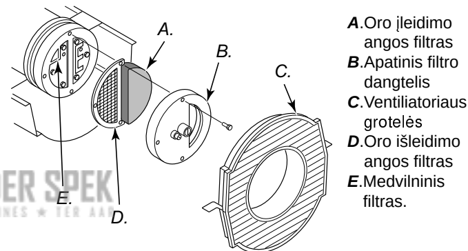
16 pav. Oro išleidimo / įleidimo angų ir medvilniniai filtrai (10 kW ir 20 kW CED modeliai).
