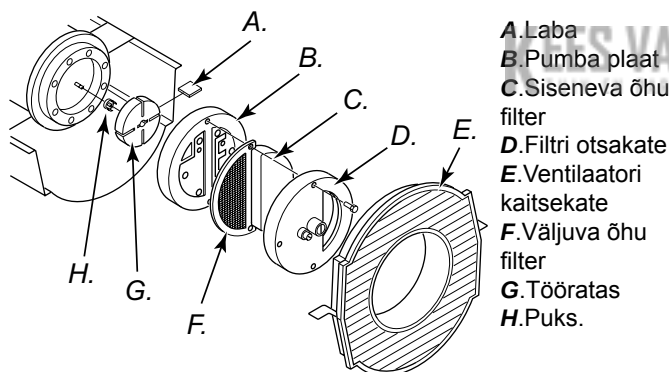
Joonis 25. Tööratta asukoht, mudelid võimsusega 10 kW ja 20 kW.
