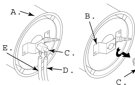
Figur 20 - Aftagning af luft- og petroleumsslang (10Kw Model)
