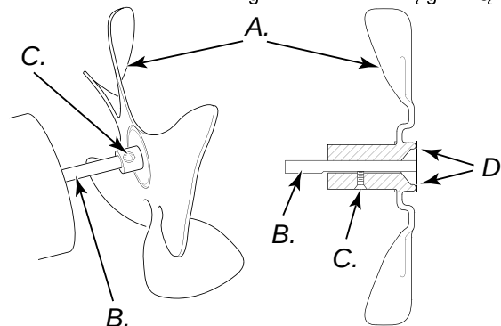
29 pav. Ventiliatoriaus, variklio veleno irkšavimo varžto išdėstymas.
