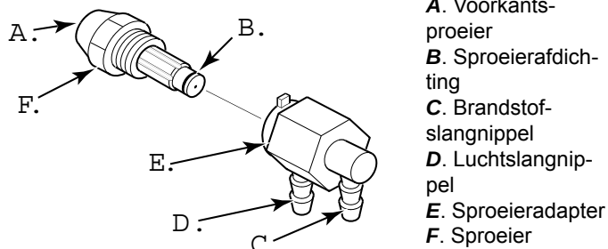
Figuur 22 – Sproeier en sproeieradapter, model 10 kW.
