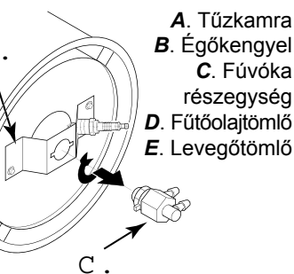
21. ábra - A fűvóka részegység leszerelése, 10 kW modell
