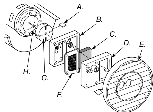
26 pav. Rotoriaus ištara (29 kW ir 44 kW CED modeliai).
