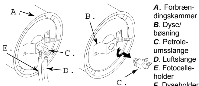
Figur 20 - Aftagning af luft- og petroleumsslang (10Kw Model) Figur 21 - Aftagning af dyse og dysetilpas.
