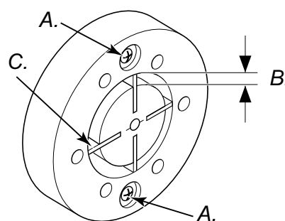
Figuur 27 – Plaats van stelschroeven speling.
