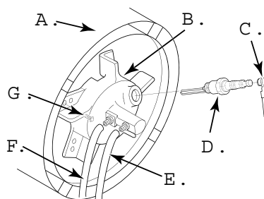
Obrázek 23 - Odmontování hlavy hořáku - Modely s vákonem 20/29/44 kW.
