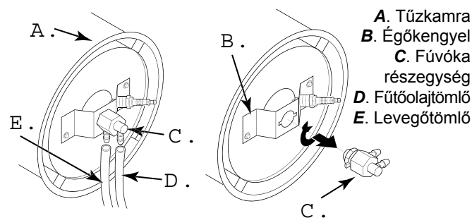
20. ábra - A levegő- és fűtőolajtömlők levétele, 10 kW modell
