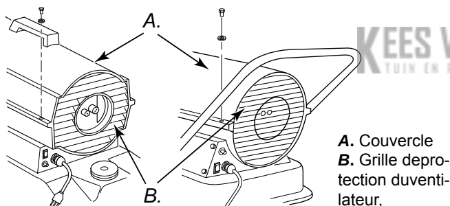
Figure 7-8 – Dépose du couvercle, Modèles.
