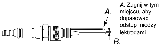
Rysunek 15 - Odstęp między elektrodami świecy zapłonowej, modele 20kW, 29kW, 44kW.
