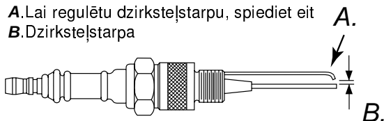
15. zīmējums - Aizdedzes sveces dzirkstelstarpā, modeļi ar jaudu 20 kW / 29 kW / 44 kW.
