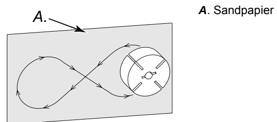
Abbildung 28 – Abschmirlen des Rotors.
