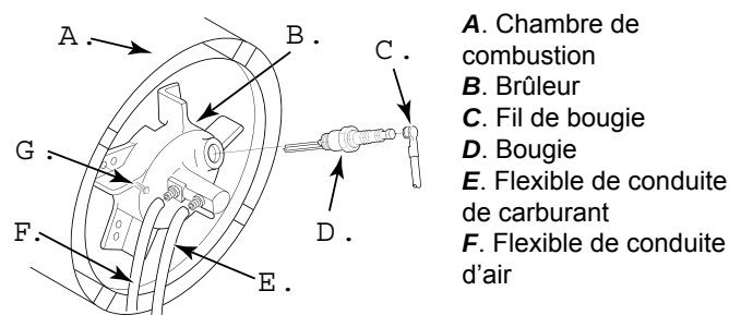
Figure 23 – Dépose du brûleur, Modèles 20, 29 et 44 kW.
