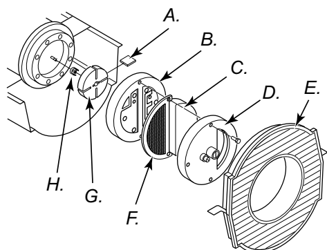
25. ábra - A forgórész elhelyezkedése, 10kW és 20kW modellek
