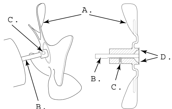
A. Lüfter, B. Motorwelle, C. Stellschraube, D. Bündig.
