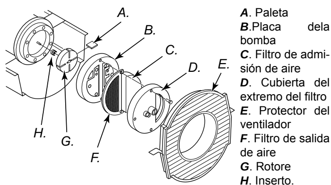
Figura 25 – Ubicación del rotor, modelos de 10 y 20kW.
