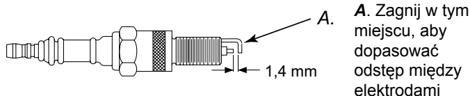
Rysunek 12 - Odstęp między elektrodami świecy zapłonowej, model 10 kW.
