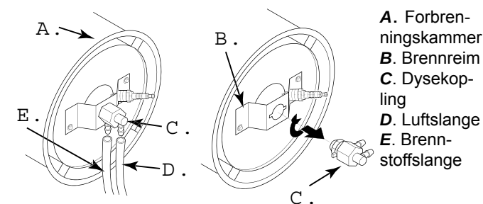
Figur 20 – Fjerning luft og brennstoffslange 10 kW Modell.
