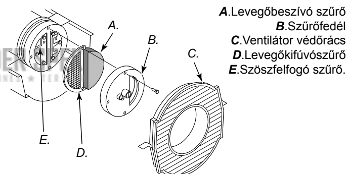
16. ábra - Levegőkifúvó-, levegőbeszívó- és szőszelfogó szűrők. 10/20 kW modellek
