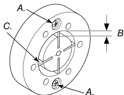
27. ábra - Hézagbeállító csavarok helye
