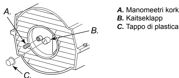
Joonis 18. Manomeetri korgi eemaldamine, mudelid võimsusega 10 kW ja 20 kW.
