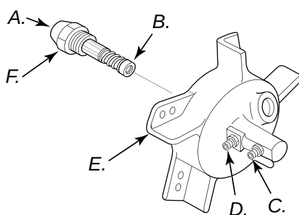
24. zīmējums – Sprauslas izņemšana, modeļi ar jaudu 20 kW, 29 kW, 44 kW.
