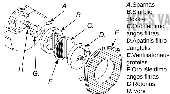
25 pav. Rotoriaus ištara (10 kW ir 20 kW CED modeliai).
