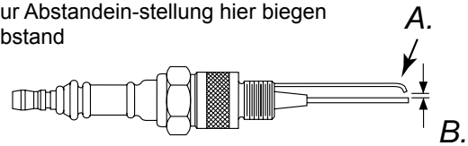
Abbildung 15 – Elektrodenabstand 20, 29, 44 kW Modelle.
