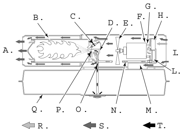
Figur 4 – Funktionsdiagram.
