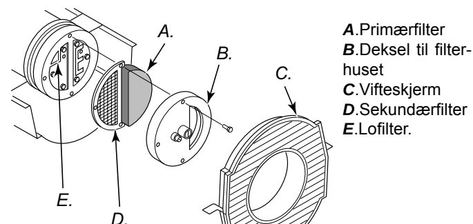
Figur 16 – Primærfilter, sekundærfilter og lofilter, modellene 10 kW og 20 kW.
