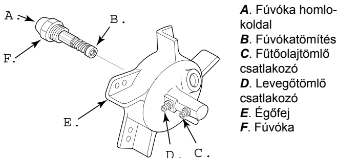
24. ábra - A fűvóka kiszerelése, 20/29/44 kW modellek
