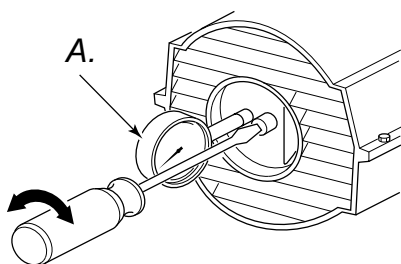
Kuva 19 – Pumpun paineen säätö.
