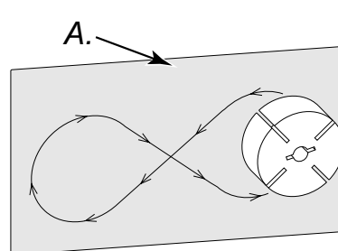
Figur 28 – Att slipa rotorn
