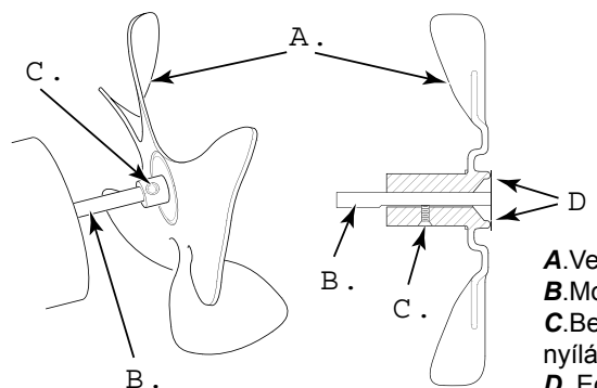
29. ábra - A ventilátor, motortengely és belső kulcsnyílású csavar elhelyezkedése
