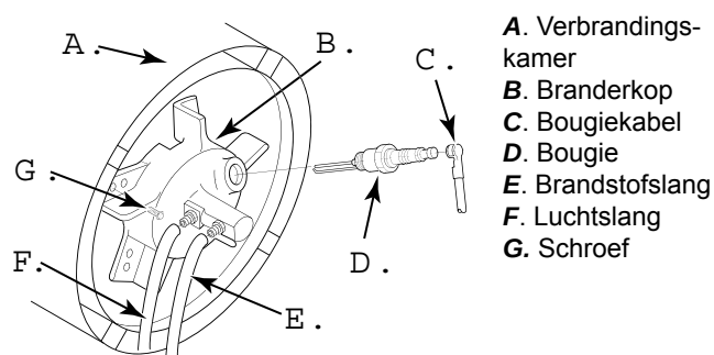
Figuur 23 – Verwijderen van branderkop, modellen 20, 29 en 44 kW.
