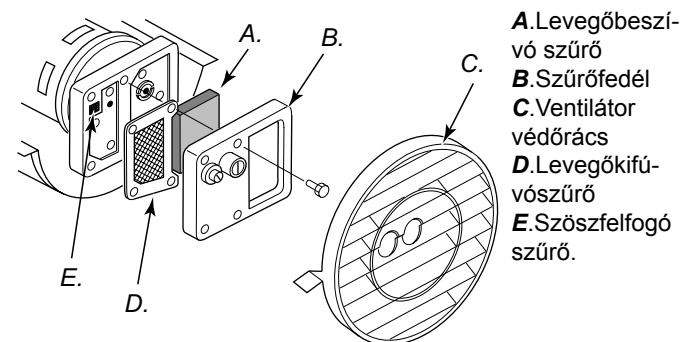
17. ábra - Levegőkifúvó-, levegőbeszívó- és szőszelfogó szűrők. 29/44 kW modellek
