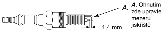
Obrázek 12 - Mezera jiskřiště svíčky - Model s vákonem 10 kW.
