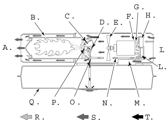
Figure 4 – Coupe, fonctionnement.
