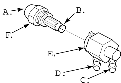
Figur 22 – Dyse og dysebøsning.
