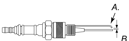
Kuva 15 – Sytytystulpan väli, malli 10 kW.
