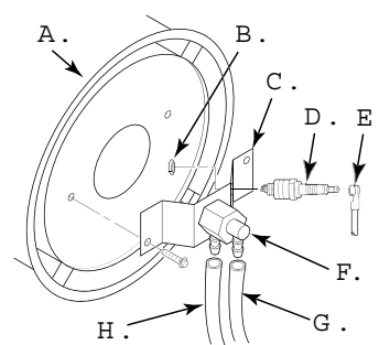
Rysunek 11 - Wyjmowanie świecy zapłonowej, model 10 kW
