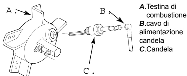
Figura 14 – Rimozione candela.
