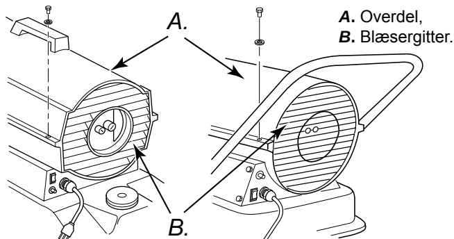
Figur 7-8 – Model 10 kW, 20 kW, 29 kW og 44 kW afmontering af overdelen.
