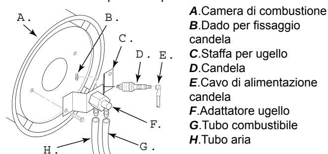
Figura 11 – Rimozione candela.
