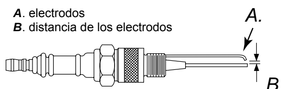
Figura 15 – distancia de los electrodos de la bujía.
