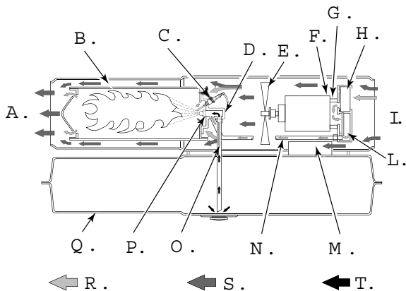
Kuva 4 – Toimintäpileikkaus.
