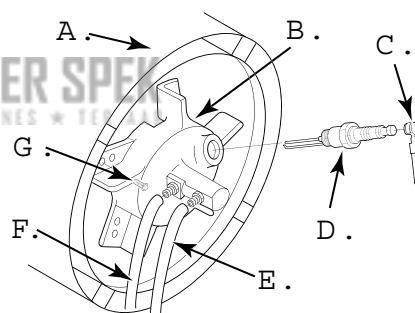
Figur 23 Fjernelse af Brndkammerhovedet, 20/29/44 kW.
