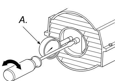
Kuva 19 – Pumpun paineen säätö.
