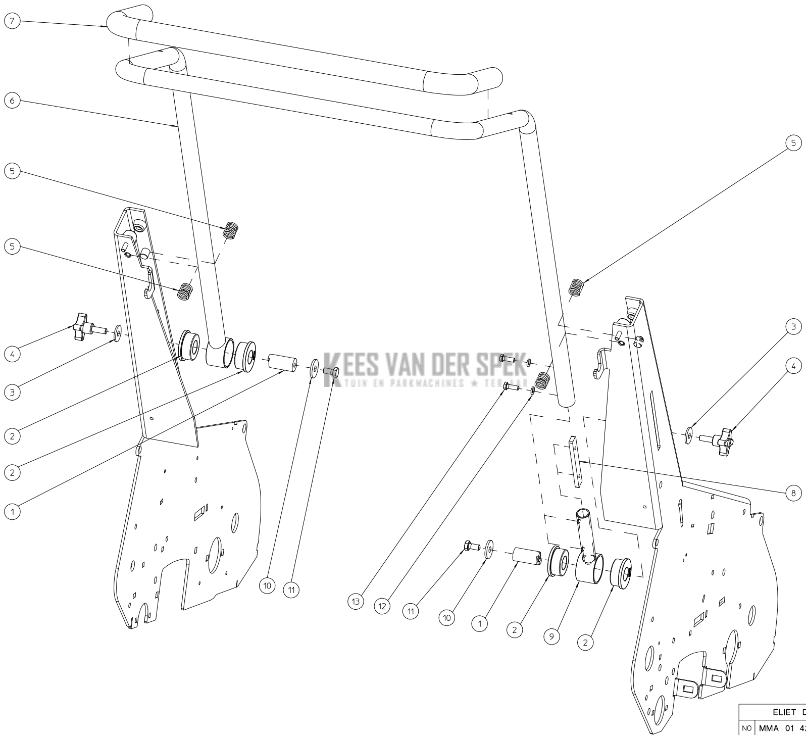
1/3-Montage Stuur
