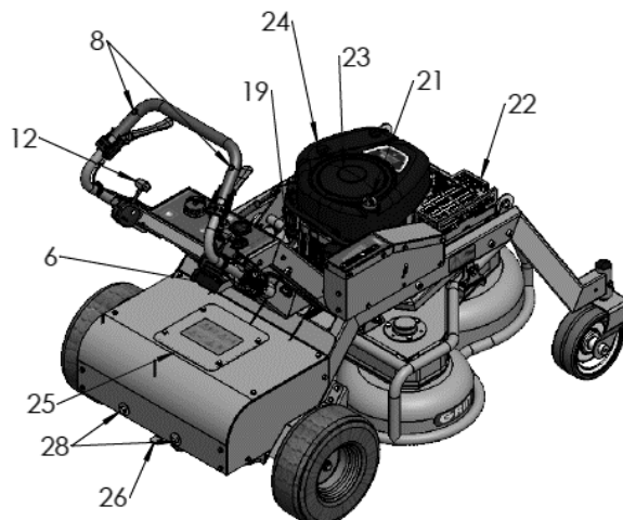
Afb. 7 - Machineonderdelen
