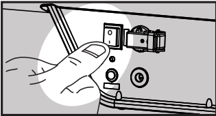
2. Stil ventilens afbryder i position I.
